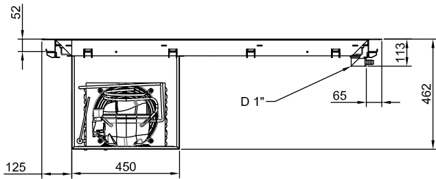
Zij aanzicht
